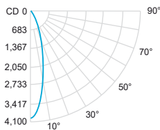
Spot 24° (3000K, 80 CRI)
